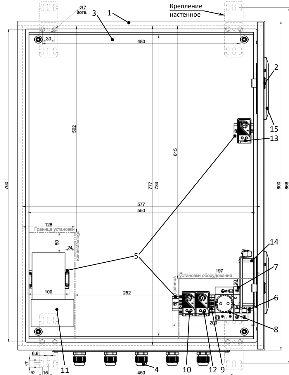
Рисунок 1 – Устройство шкафа
