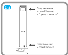
06 Подключение к сети Ethernet и "сухие контакты".
