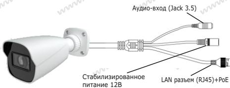
Рис.1 Схема подключения
