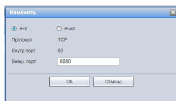
Рисунок 7.60 – Подпункт меню «UPnP»: Изменение перенаправления портов
