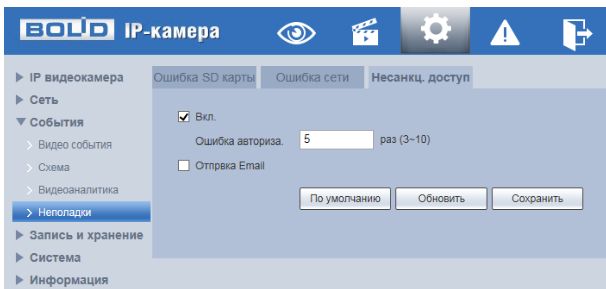
Рисунок 7.86 – Вкладка «Несанкционированный доступ»
