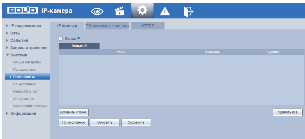
Рисунок 7.110 – Вкладка «IP Фильтр»
