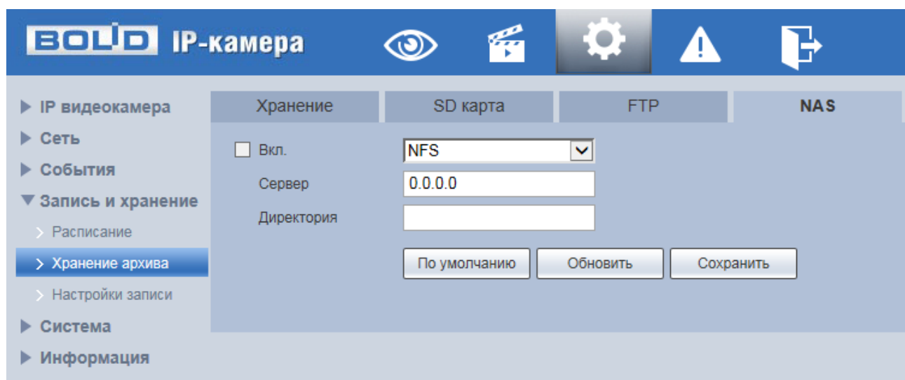
Рисунок 7.99 – Вкладка «NAS»
