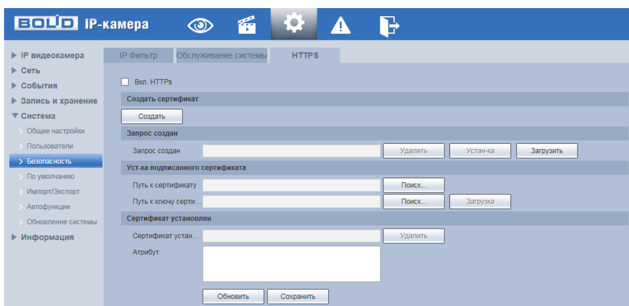
Рисунок 7.113 – Вкладка «HTTPS»
