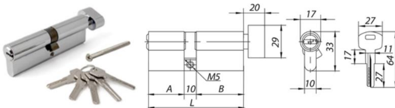
Размерный ряд цилиндров серии 500ZP
